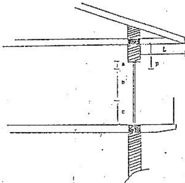
Schema esplicativo superficie illuminante utile
