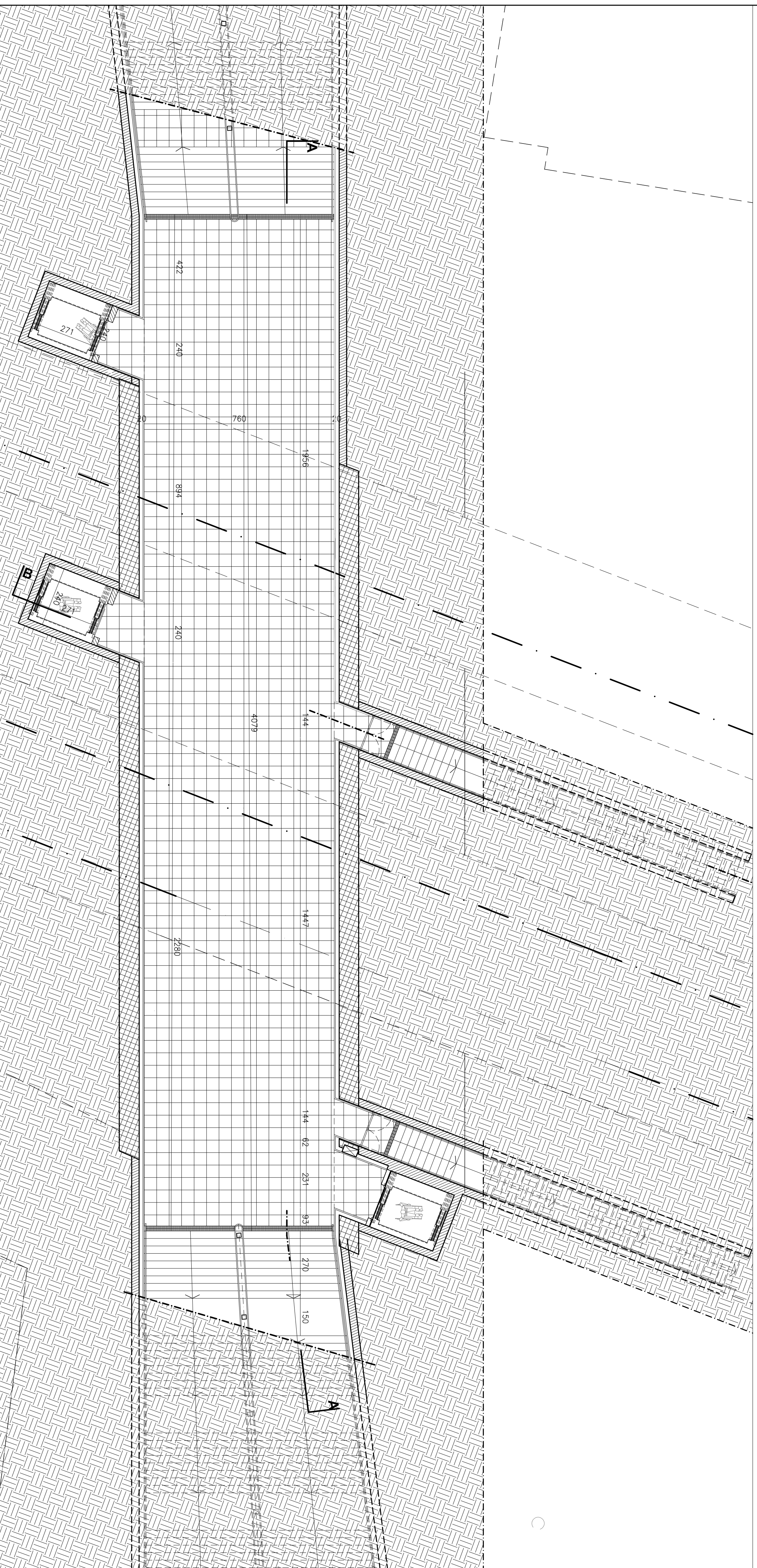
PIANTA SOTTOPASSO DI STAZIONE QUOTA + 144.33
